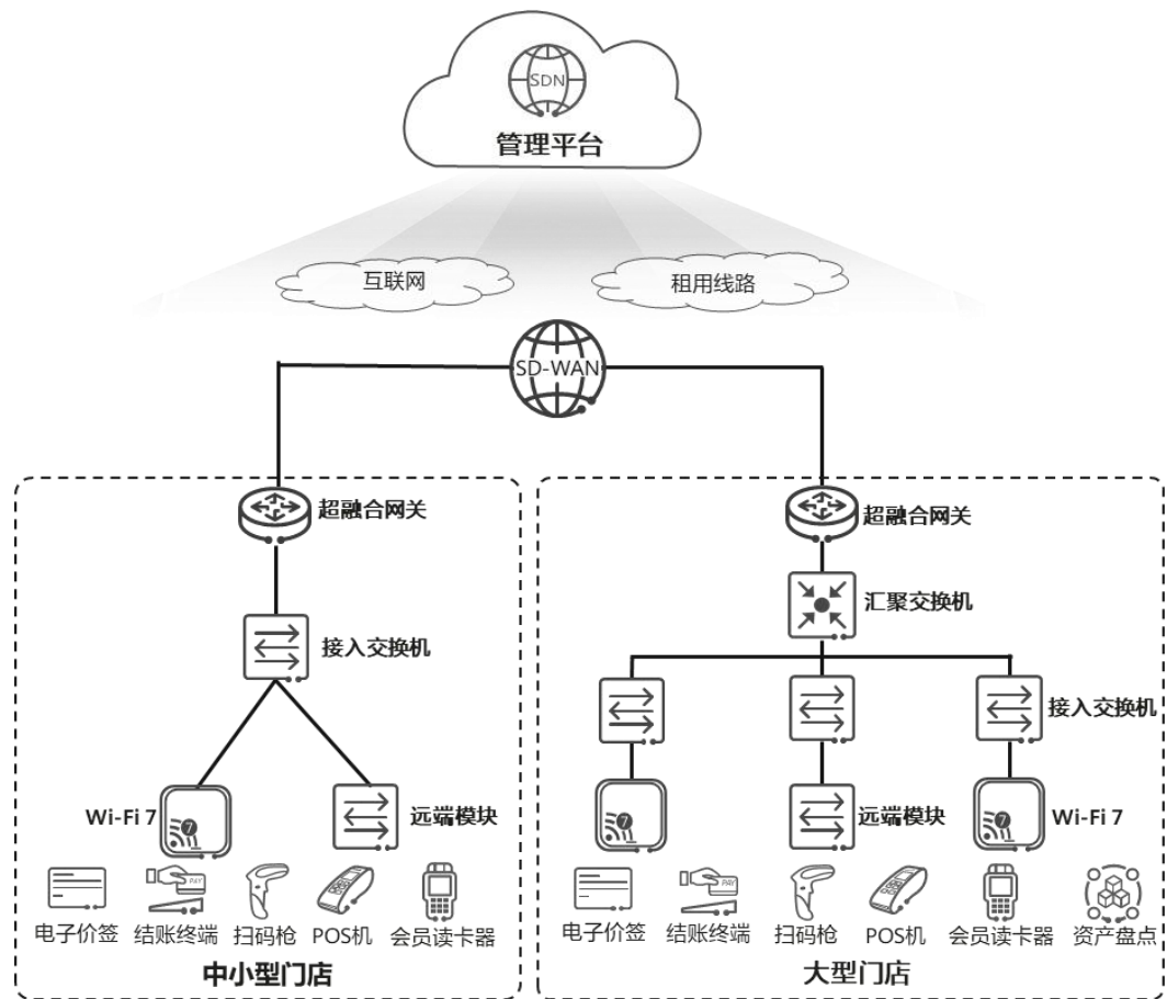
图 3-6 推荐组网架构
