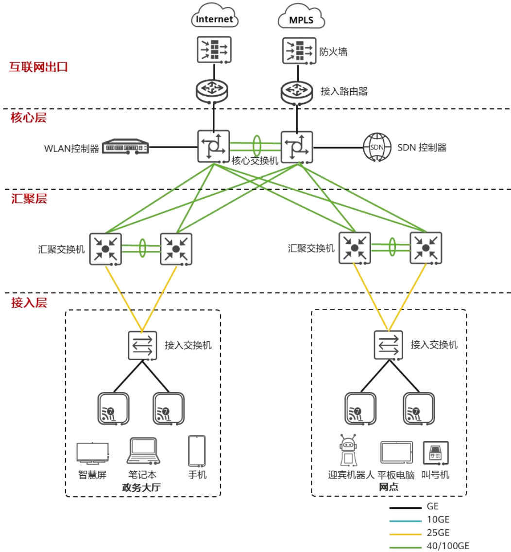
图 3-3 推荐组网架构
