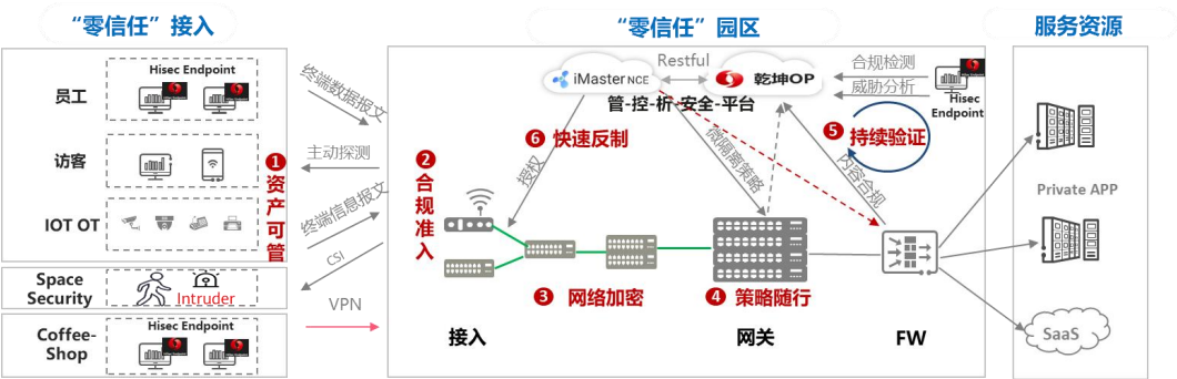
图 2-16 园区网络安全架构
