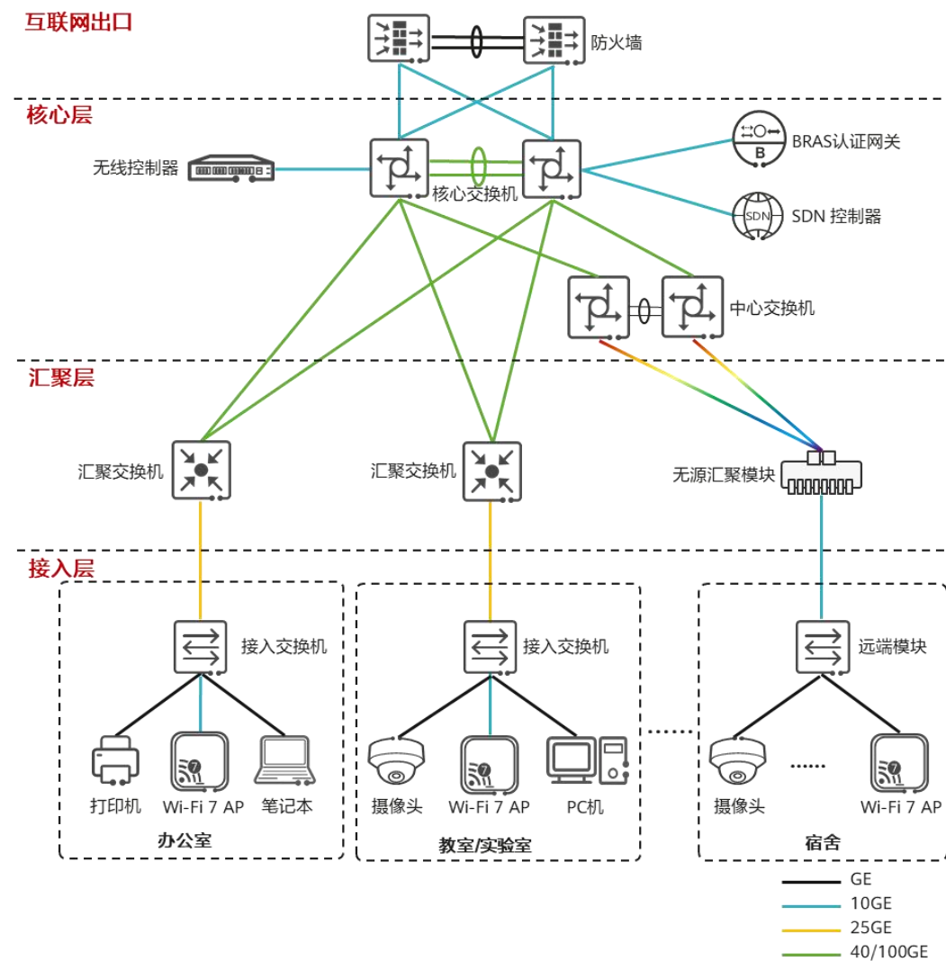
图 3-1 推荐组网架构
