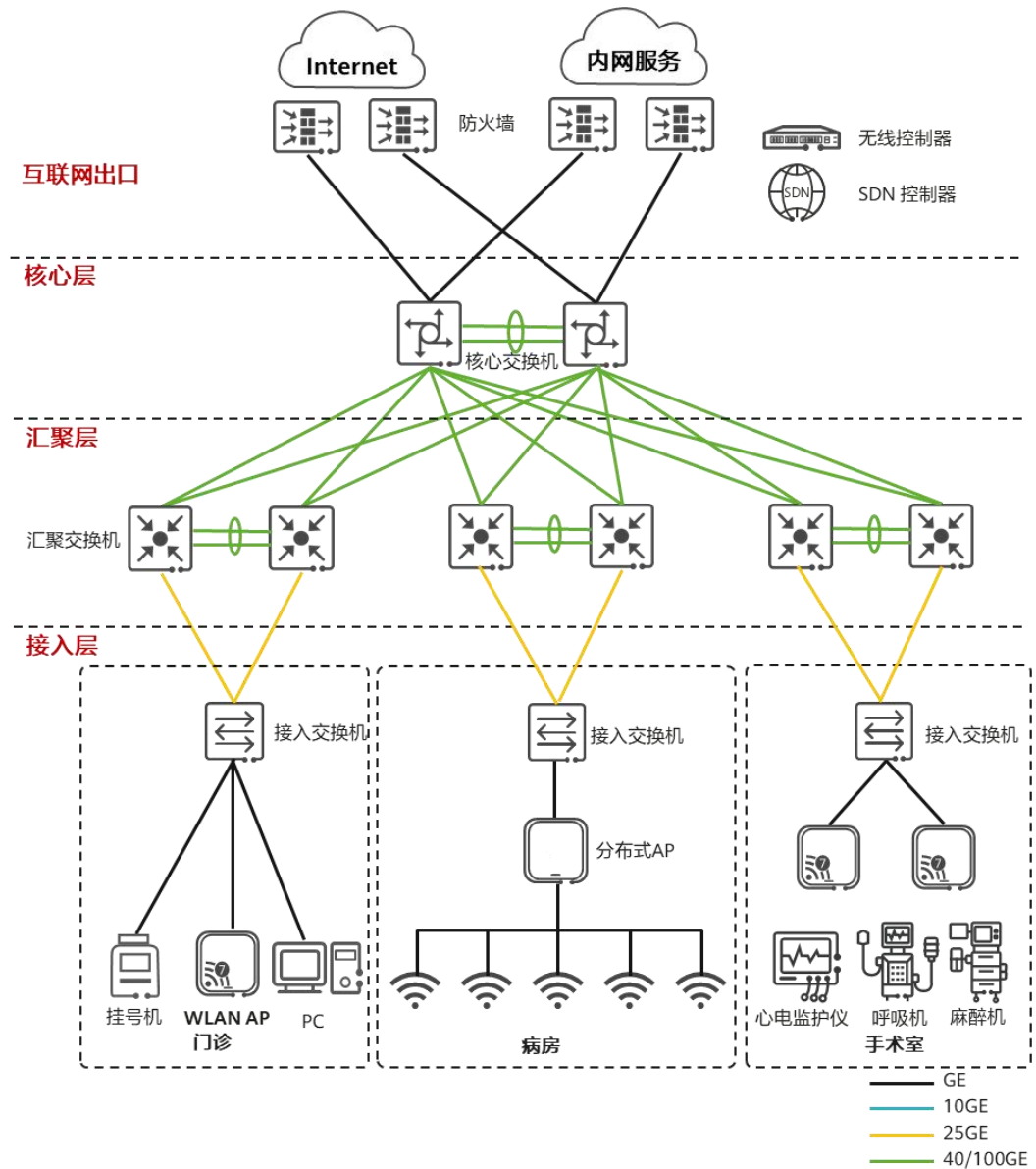
图 3-4 推荐组网架构
