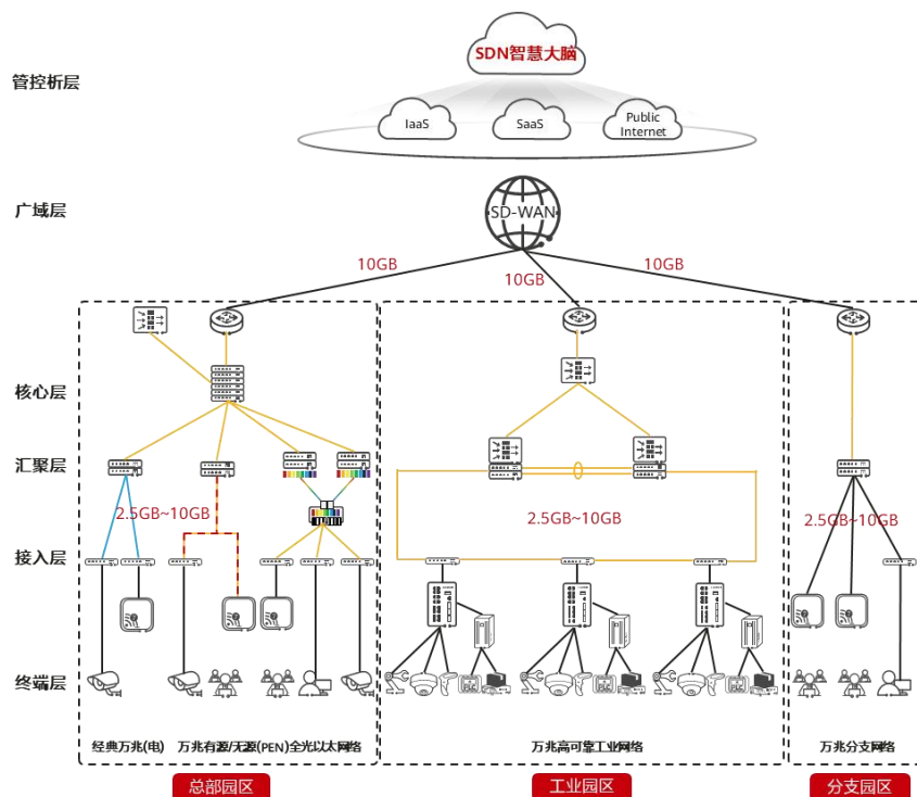
图 2-1 高品质万兆园区网络物理架构
