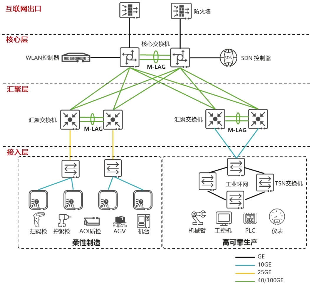
图 3-5 推荐组网架构
