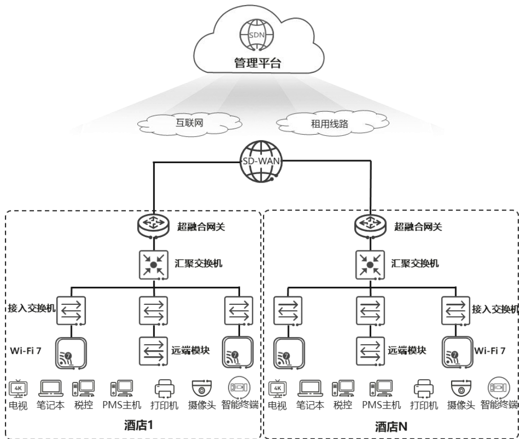
图 3-7 推荐组网架构
