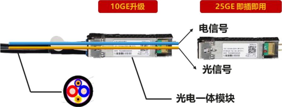
图 2-9 光电混合电缆和光模块构成
