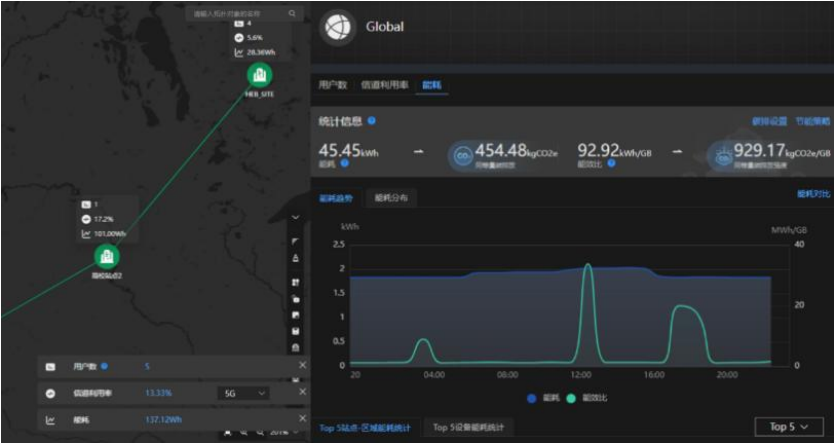
图 2-15 WLAN 网络可视化系统园区能耗监控
