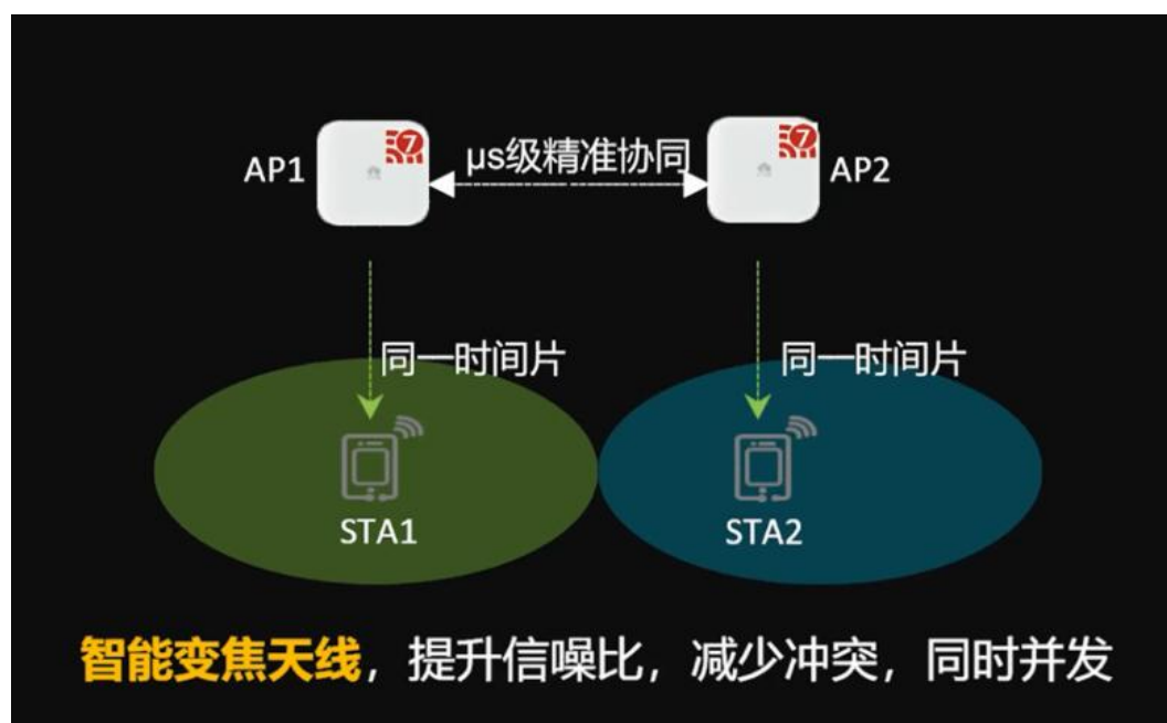
图 2-10 智能天线和多 AP 协同工作示意图
