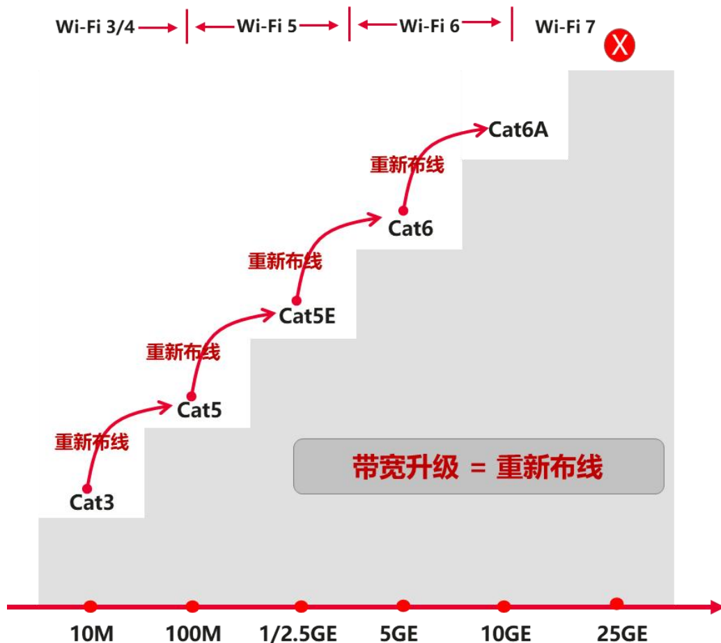
图 2-5 电缆与 Wi-Fi 代际演进关系
