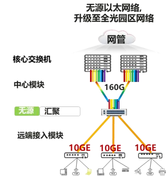
图 2-8 极简无源 10GE 全光网络
