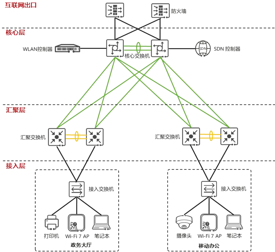
图 3-2 推荐组网架构
