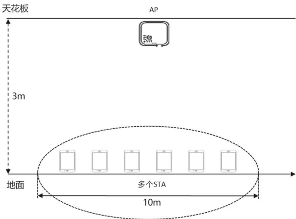
图7 单频段多用户并发吞吐场景模型
