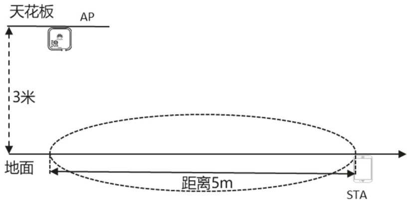
图10 单用户 5m 无遮挡性能场景模型
