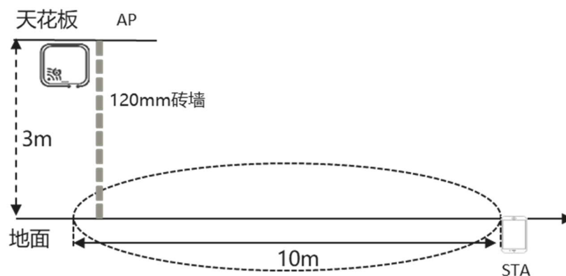
图9 单用户 10m 视距穿墙性能场景模型
