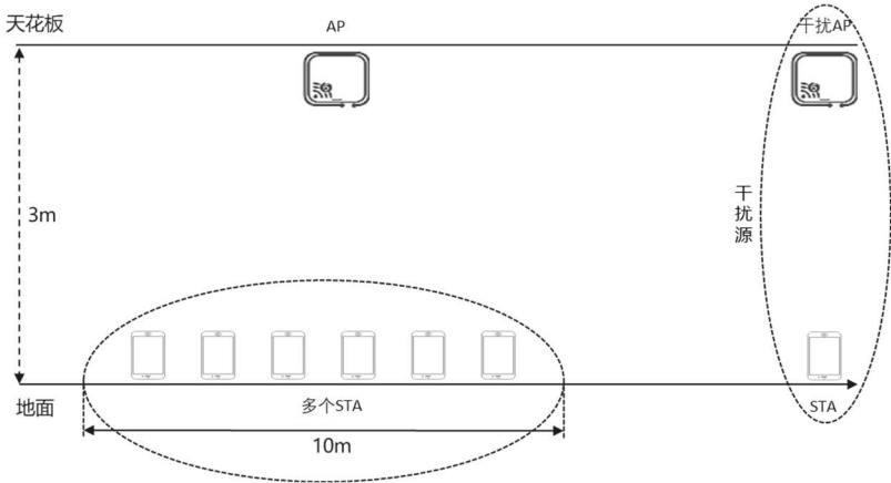
图14 干扰条件下多用户并发时延场景模型
